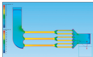
Přehledné znázornění rozložení tlaků (vlevo) a rychlostí (uprostřed). Náběhové koleno vlevo i bez vodicích plechů zajišťují rovnoměrné zaplavení všech komor tlumiče. Vpravo je rozložení rychlostí ve výstupním kolenu tlumiče. Snímky poskytla společnost Greif-akustika
