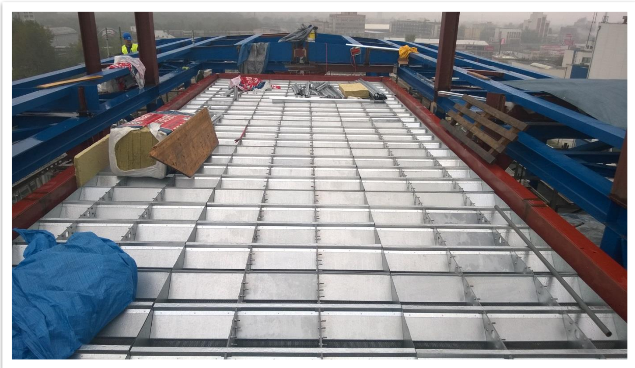
Montáž nosného rámu.
